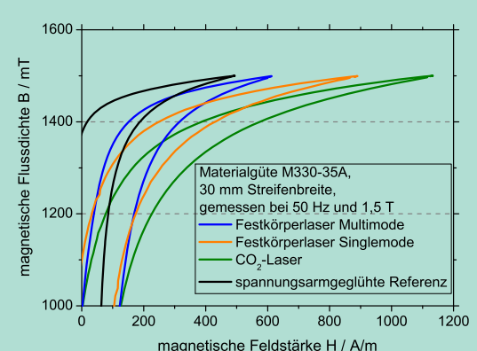
Die Wahl der Strahlquelle beeinflusst den Eigenspannungszustand der Probe (Ausschnitt der Hysteresekurve)
