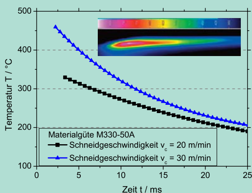
Bestimmung des zeitlichen Temperaturprofils in einem festen Punkt mit konstantem Abstand von 100 µm zur Schnittkante
